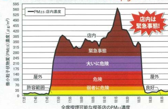
■タバコの吸える喫茶店のPM 2.5 は371μg/m 3 (平均値)
